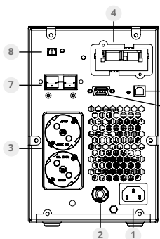
Задняя панель ИБП ФОРА 1000/1500
