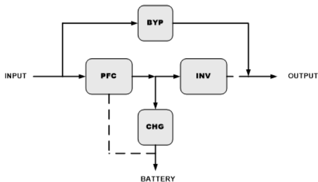
Рисунок 4.4. Эко-режим
