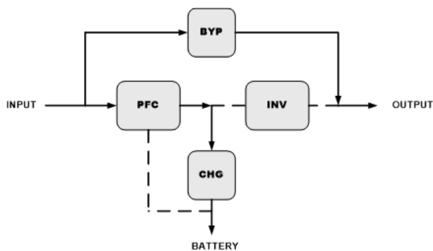
Рисунок 4.2. Режим байпаса
